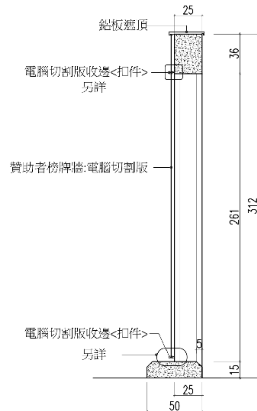
3 羅馬框牆剖面圖 W-07 Scale: 1/30cm
