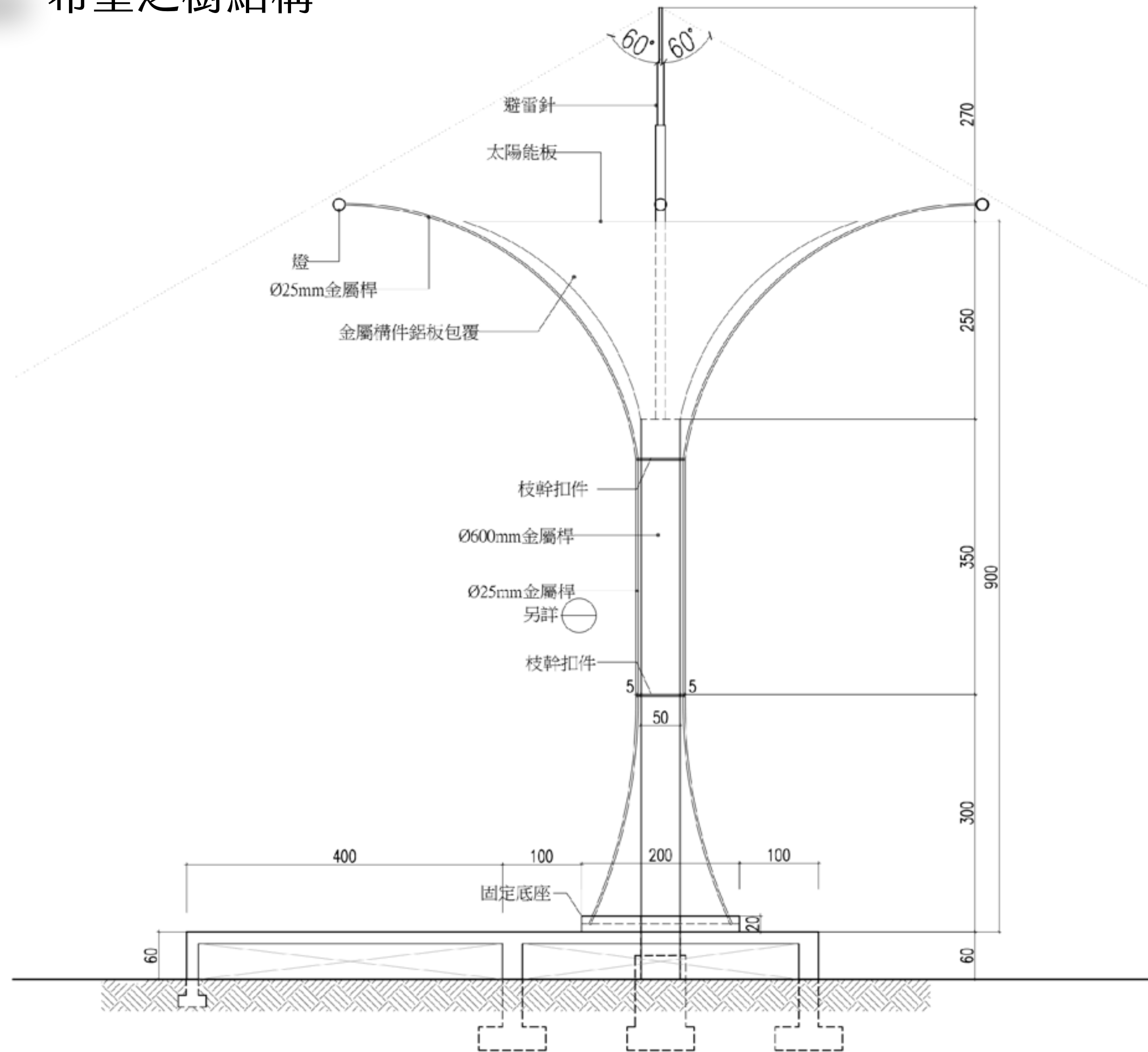
1 希望之樹剖面圖 W-05 Scale:1/60cm
