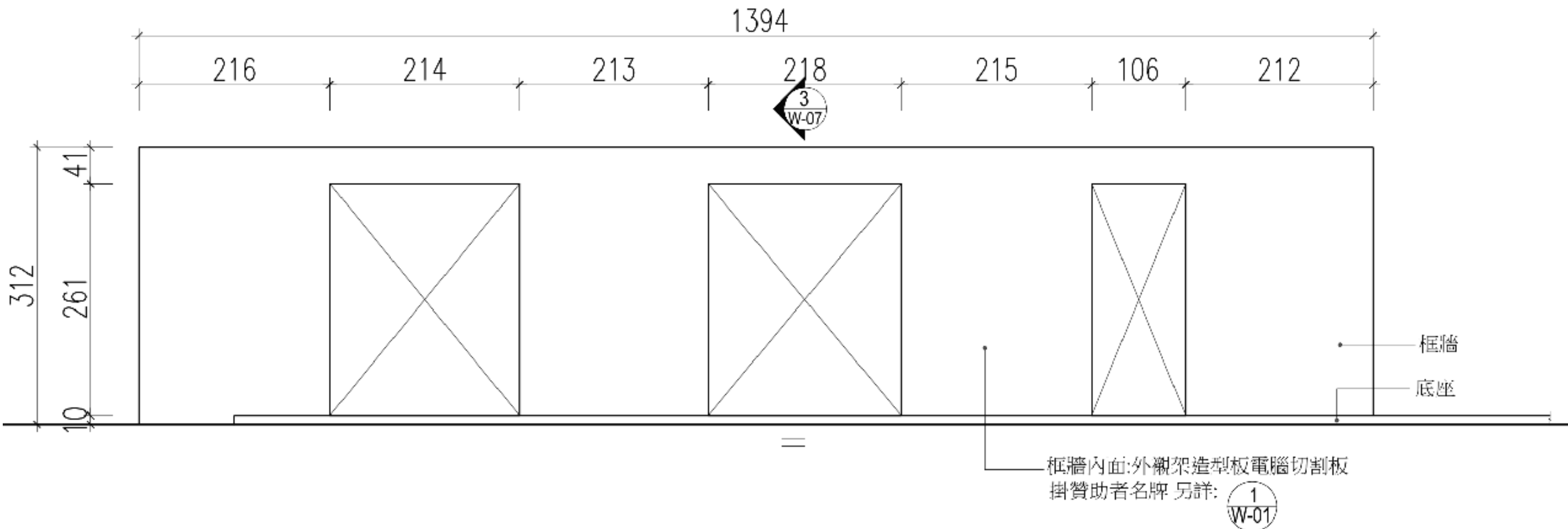
2 羅馬框牆展開立面圖 <現況> W-07 Scale: 1/60cm
