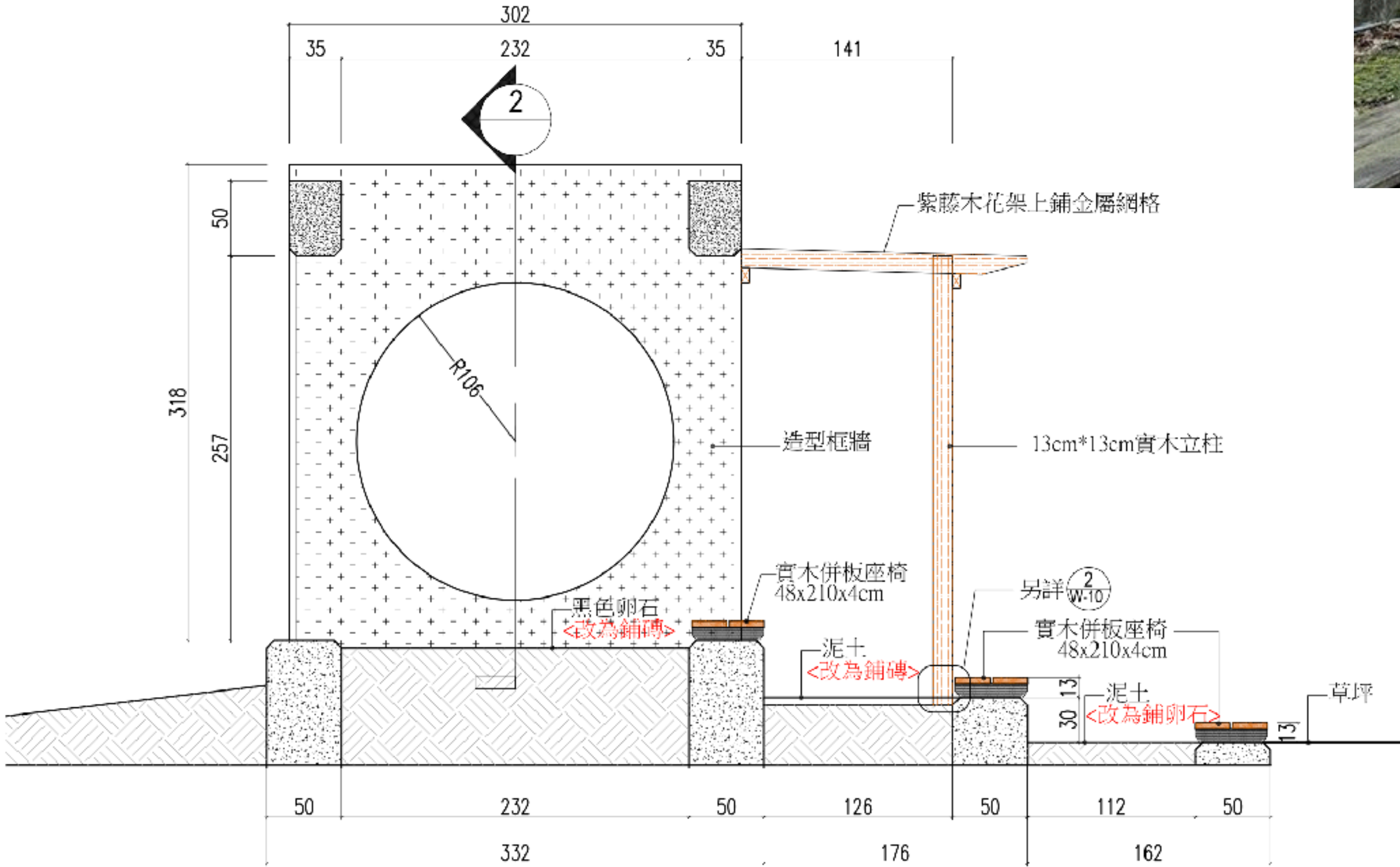
1 紫藤框牆剖立面圖 <現況> W-09 Scale:1/40 cm
